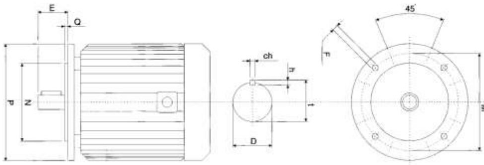
Dati tecnici motori / Technical data of motors
